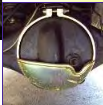
Coquille de pont à boulonner 5 mm: Avant: Defender tous modèles Arrière: Defender 90 sauf 110/130. Avant et arrière: Disco 200/300 TDI, RR classic - Réf: 1018
