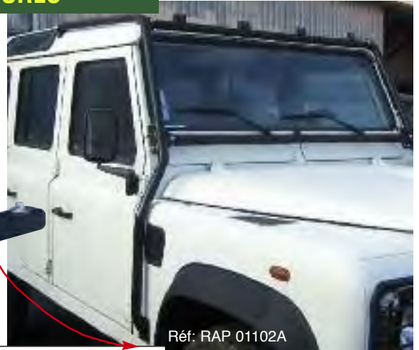
ARCEAU DE SÉCURITÉ Avec supports phares fixations de chassis et visserie pour loisirs Baie de pare-brise: 90/110/130 Réf: RAP 01102A Arceau 6 points Def 90 Réf: RAP 01107 Arceau 6 points Def 110 Réf: RAP 02102
